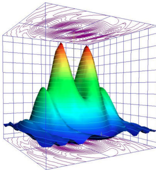
FIGURE 1 – Représentation de la fonction f : \mathbb{R}^2 \mapsto \mathbb{R} définie par (x, y) \mapsto z = \frac{\sin(x^2+3y^2)}{0.1+r^2} + (x^2 + 5y^2) \cdot \frac{\exp(1-r^2)}{2} , avec r = \sqrt{x^2 + y^2} , et projection des courbes de niveau sur les plans z = 0 et z = 9 .
